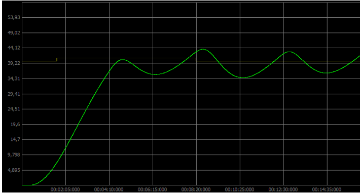
Wykres 14: Przebieg wartości regulowanej dla d = \pm 0,0001 .
