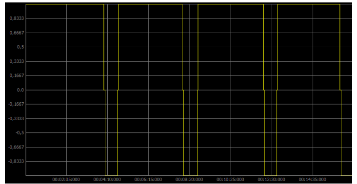
Wykres 15: Sygnał wyjściowy elementu wykonawczego.
