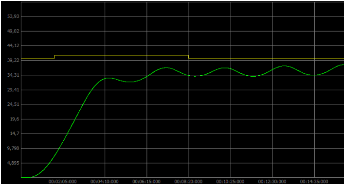
Wykres 22: Przebieg wartości regulowanej dla d = \pm 0,005 .
